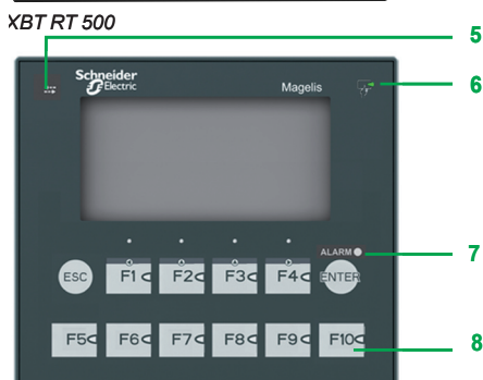
XBT RT511
