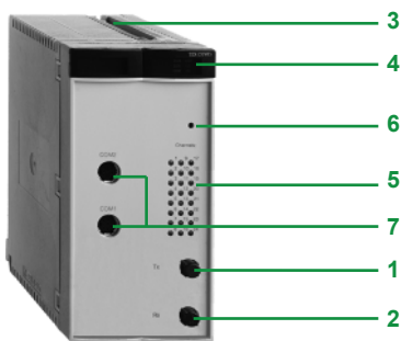
TSX CSY 85
