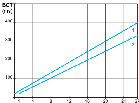
1 = 9.6 Kbps 2 = 19.2 Kbps
