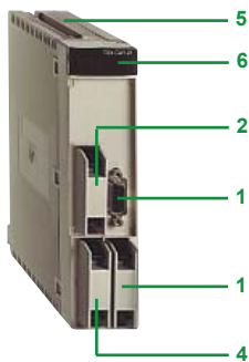
TSX CCY 1128
