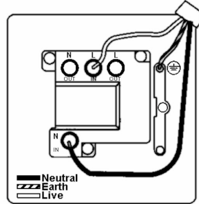
Wiring
