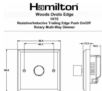
Dimensions
