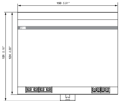
CP-T 24/20.0, CP-T 48/10.0
