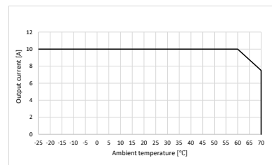
CP-S.1 24/10.0
