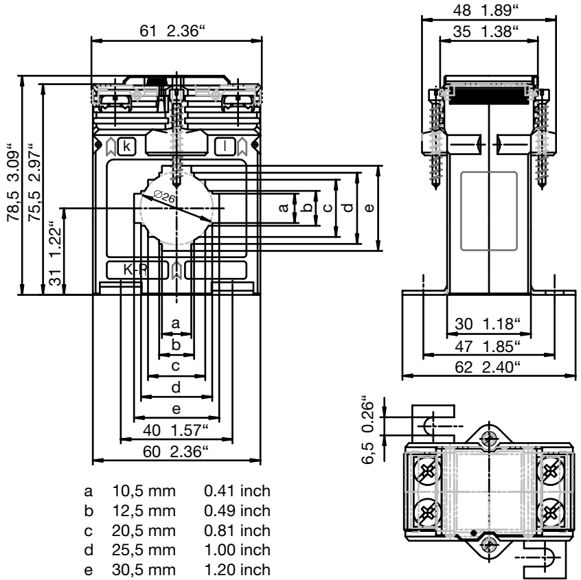
CM-CT
