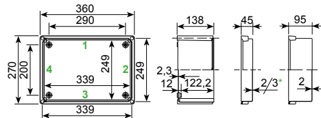
NSYPLS●●●2736G
