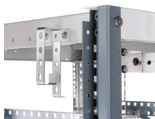
NSYGC1010
