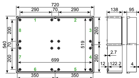
NSYPLS●●●5472G
