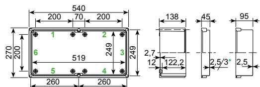
NSYPLS●●●2754G
