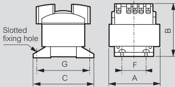
Fig. 1 - 40 to 220 VA
