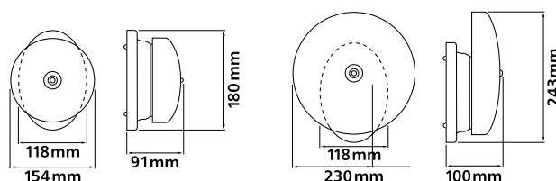
DIMENSIONS
